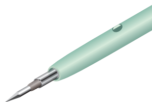
Obturator mit Trokarkanüle und Pigtail-Katheter in montiertem Zustand obturator with trocar cannula and pigtail catheter in assembled condition
